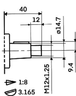
Z5 1:8 Taper Shaft
